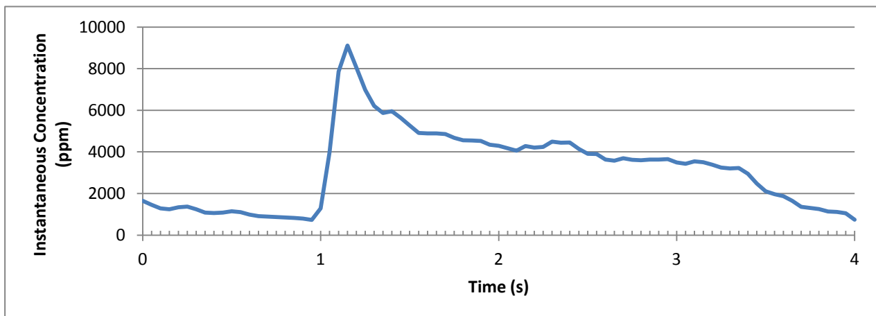
SprintIR™ Sensor
